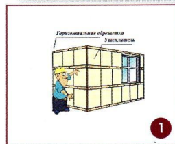
Монтаж плитки на бревенчатую стену
