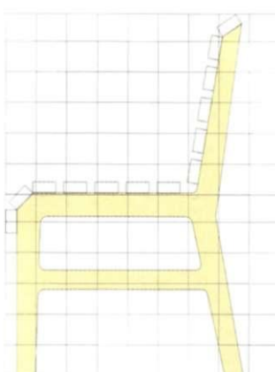
▼ Шаблон для выпиливания боковых опор
